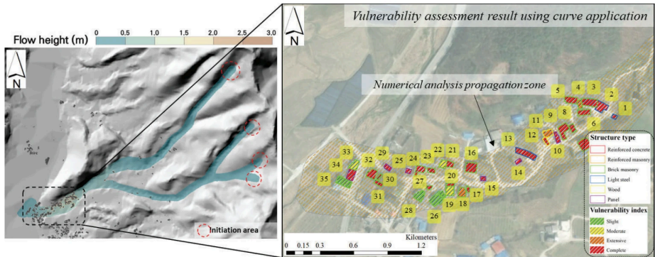
그림 4 건물 형식에 따른 취약곡선 적용
