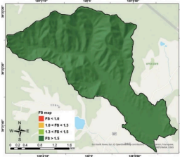
(a) 산불 발생 전(점착력 100%)
