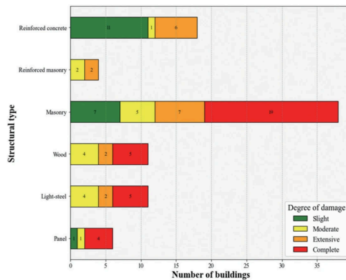
그림 2 토사재해로 피해받은 건물 분석
