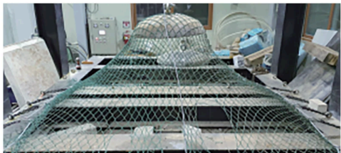
망편침시험 (상지대학교)
