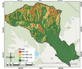
(c) 산불 발생 후(점착력 25%)
