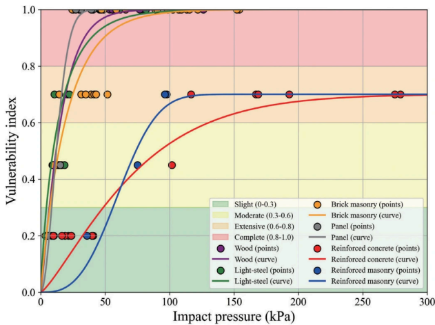
그림 3 건물 형식에 따른 취약곡선
