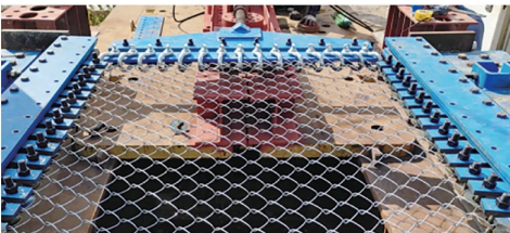
망장력 공인성능시험 (한국건설시험원)
